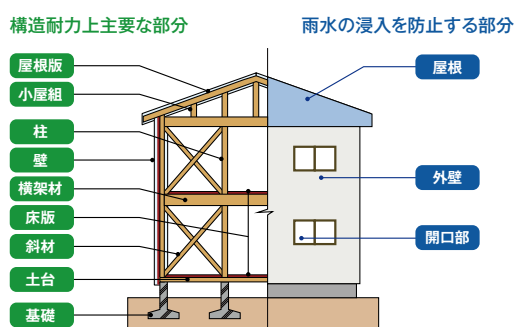
木造(軸組工法)住宅の例
