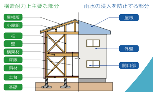
木造（軸組工法）住宅の例
