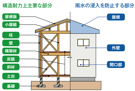
木造(軸組工法)住宅の例
