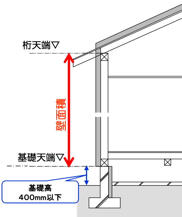
基礎断熱 + 屋根断熱
